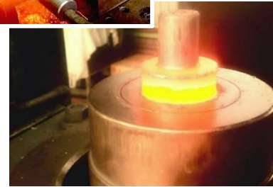
据え込みの様子(左上写真)と型打ちの様子(右下写真)
